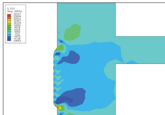
Calcul de la contrainte radiale résiduelle
