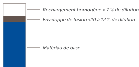
Représentation schématique d'une section transversale
