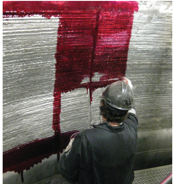
Inspección PT del recargue con soldadura
