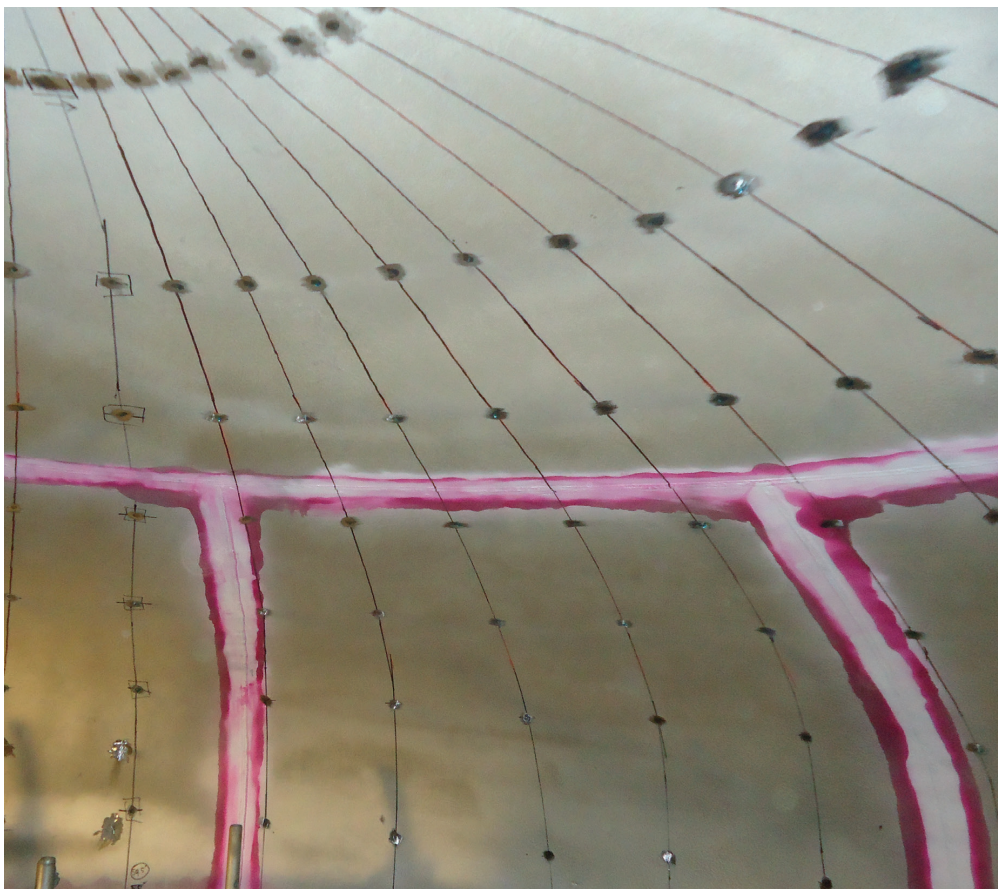
Farbeindringprüfung
