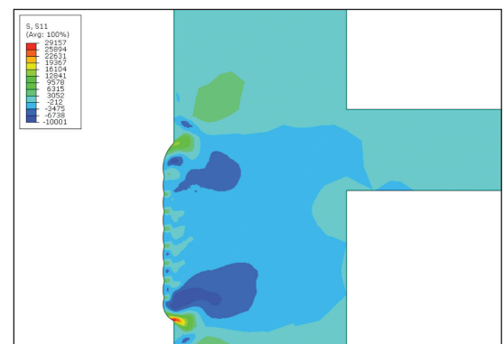
Prognose radialer Schweißeigenspannung
