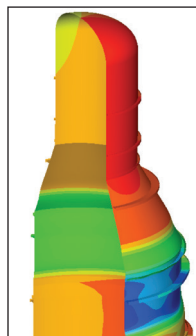
Der schattierte Bereich der Vakuumsäule zeigt die vorausberechnete Schweißschumpfung des Durchmessers an
