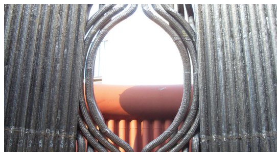
Tubi a spirale con finestre
