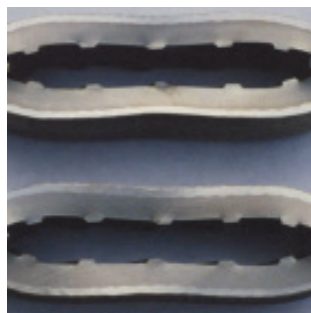
Test di appiattimento
