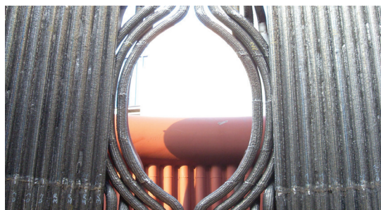
Tubes Unifuse 360 pour ouvertures
