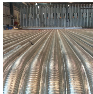
Panneau fabriqué avec des tubes Unifuse 360
