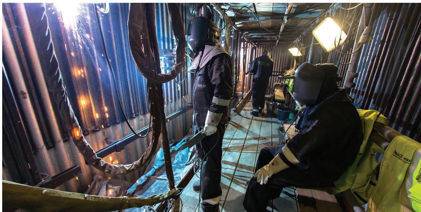
Réparation d'un mur d'eau dans une usine d'incinération
