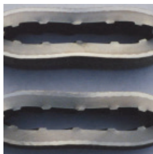
Essai d'écrasement
